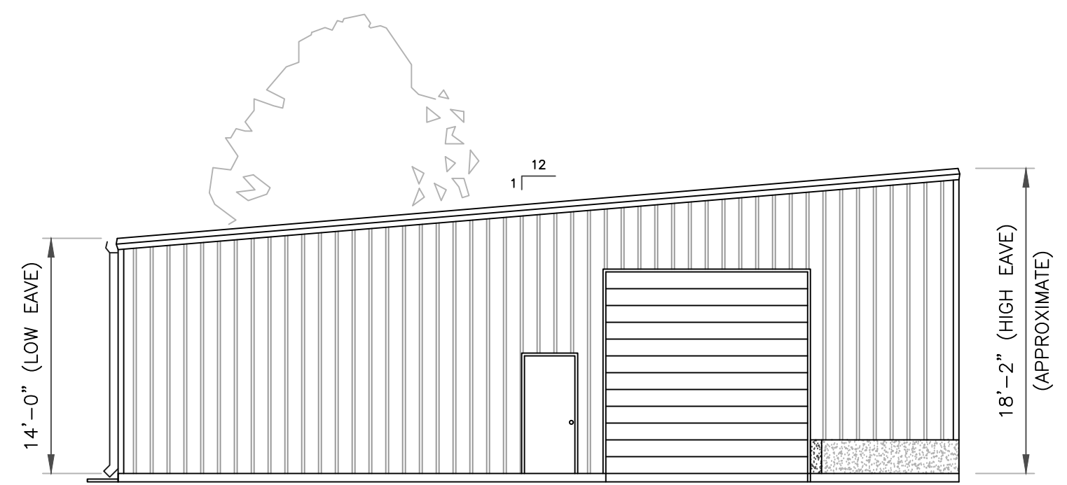
1 EAST ELEVATION SCALE: 1/8" = 1'-0"
