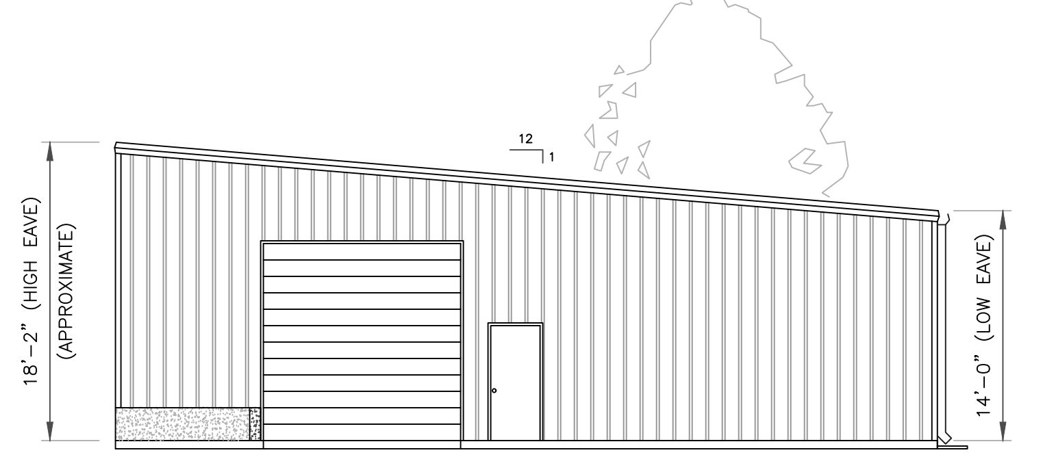
2 WEST ELEVATION SCALE: 1/8" = 1'-0"
